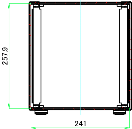
A-A ( 1 : 5.5 )
