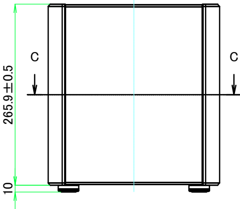
A-A ( 1 : 5.5 )
