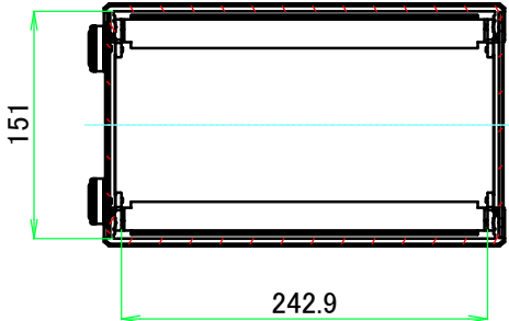
B-B ( 1 : 5.5 )
