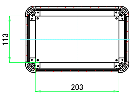
C-C ( 1 : 5.5 )
